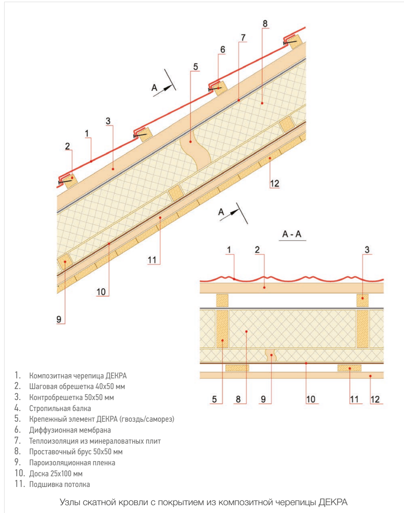
Узел 1. Состав кровли. Утепленная мансарда. Вариант 1
