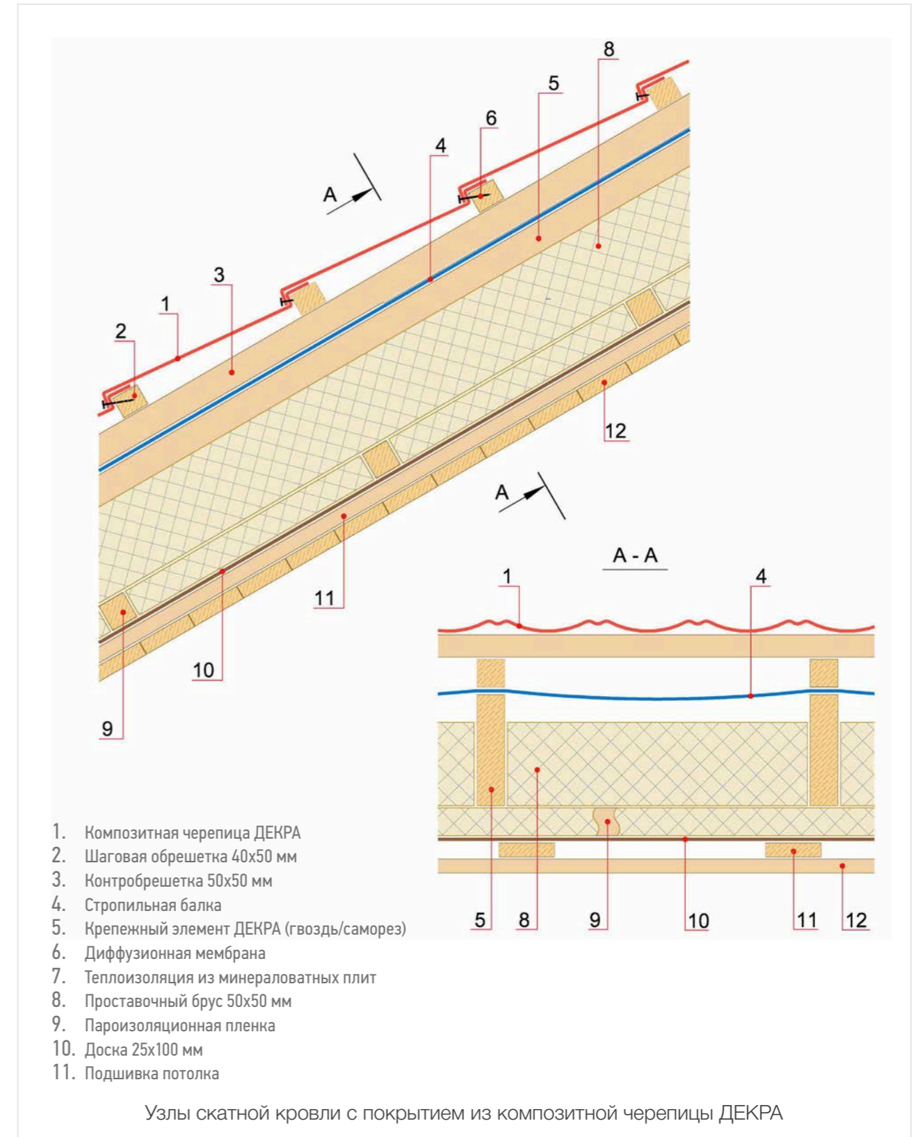
Узел 3. Состав кровли. Утепленная мансарда. Вариант 2
